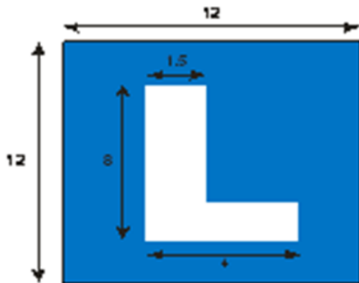
Fig.1 Tabela ndriçuese për automjete / Lighting board for vehicles / Rasvjetna tabla za vozila
