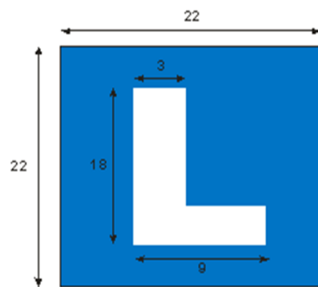
Fig.1 Tabela ndriçuese për automjete / Lighting board for vehicles / Rasvjetna tabla za vozila
